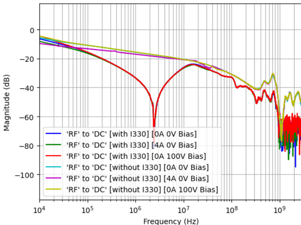
Isolation 'RF' to 'DC'
